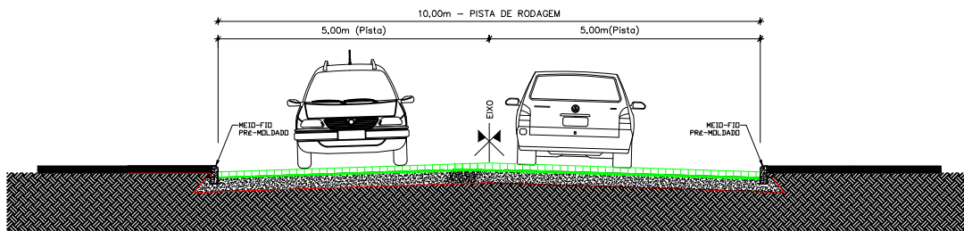
SEÇÃO TIPO DE BLOCO INTERTRAVADO - RUA JOSÉ ALOYSIO JACOBS
